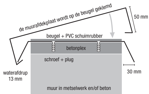
bevestigingsprincipe
